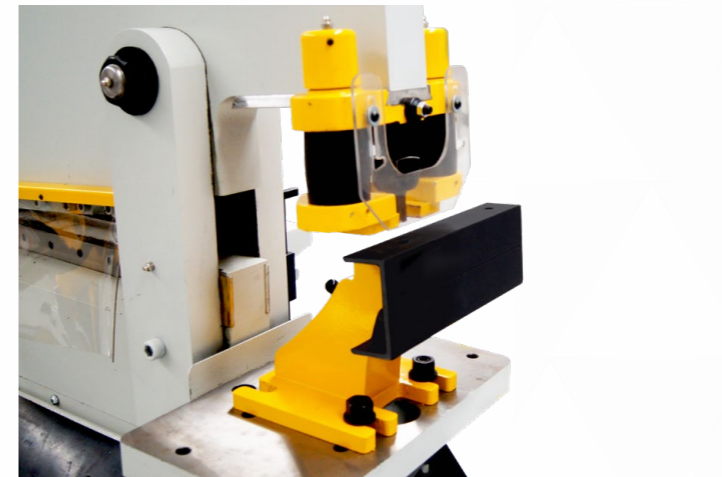
Portadados tipo cuello de ganso para punzonado de alas en canales
