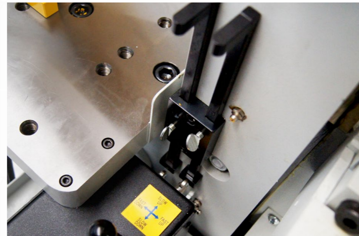
Sensores de límite electrónicos para ajuste de viaje
