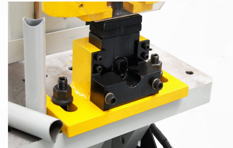
Herramental para escotar tubo
