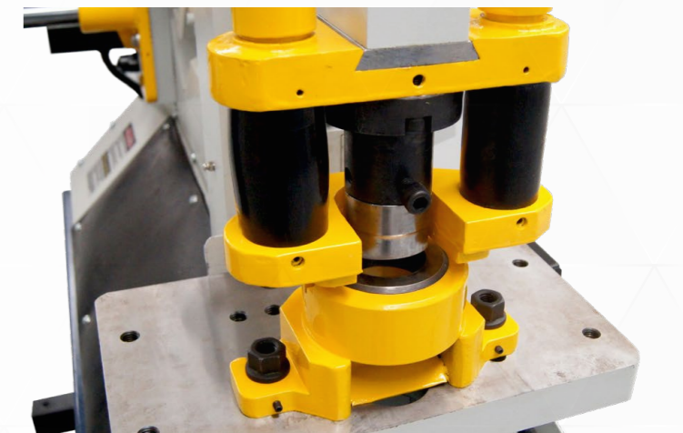
Herramental 28XX para punzonar diámetros de hasta 5"
