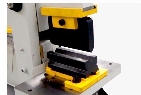
Herramental para doblado con dado inferior de 4 V
