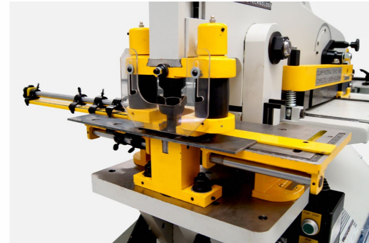
Mesa de reposicionado rápido con topes abatibles (escantillones) para punzonar agujeros múltiples en solera
